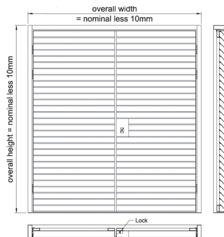
Double door
