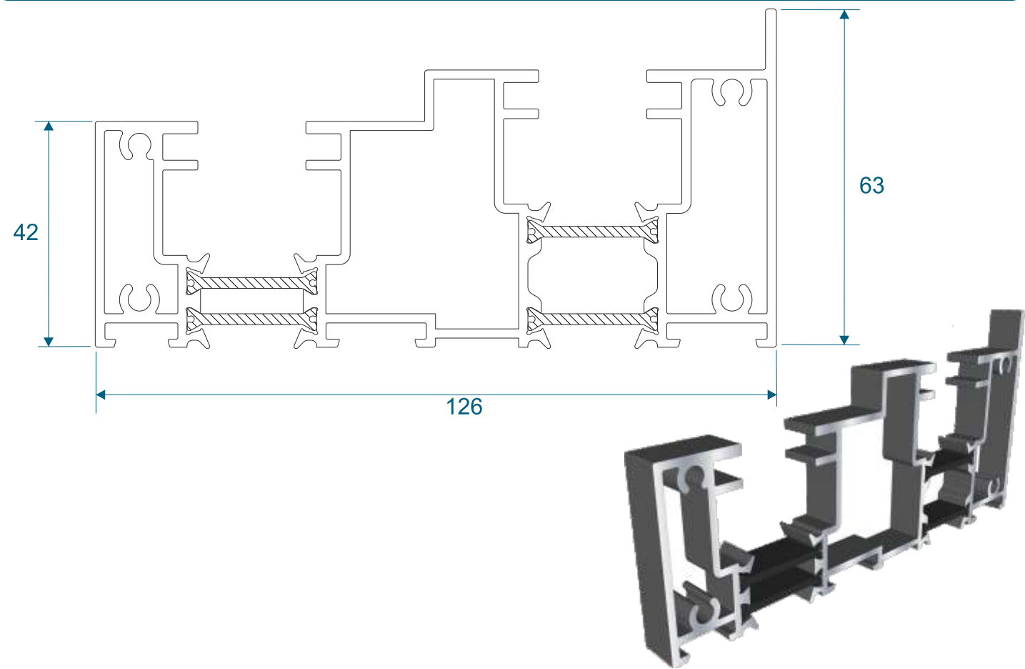
VS112 - Slim Jamb
