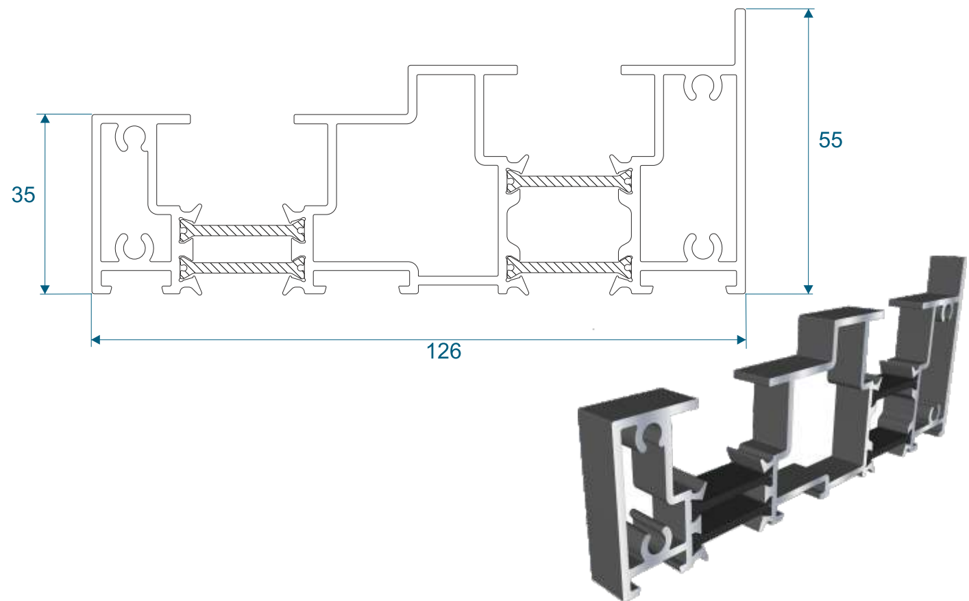
VS112 - Slim Jamb
