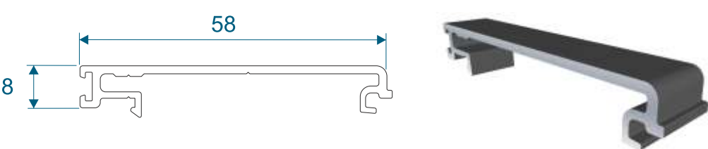
VS030 - Interlock Cap
